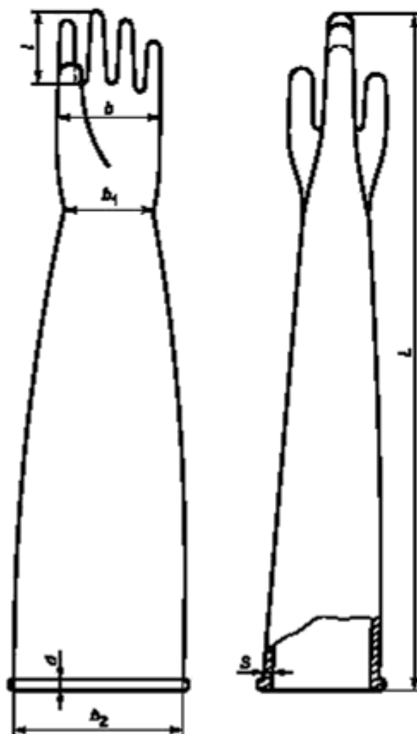
Рисунок Б.2 — Шестипалая перчатка
