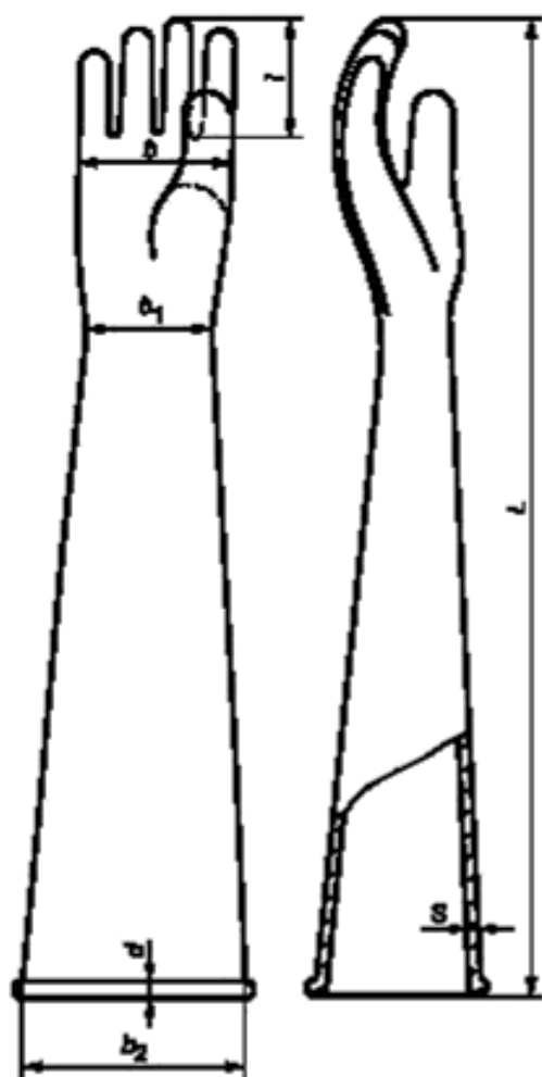
Рисунок Б.1 — Пятипалая перчатка
